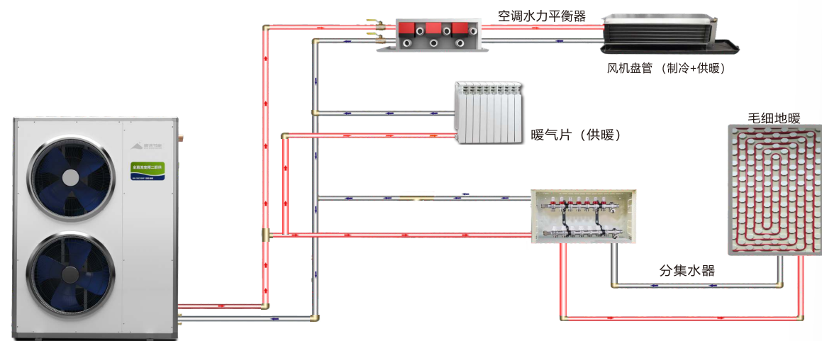
碧涞户式供暖一体机安装示意图
