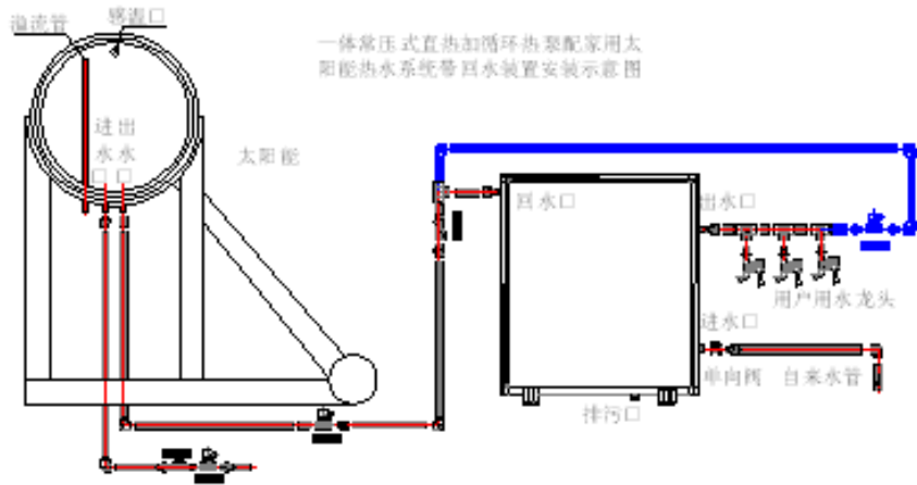
家用一体机与太阳能安装管道连接简图一：
