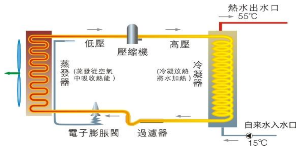
原理简图
