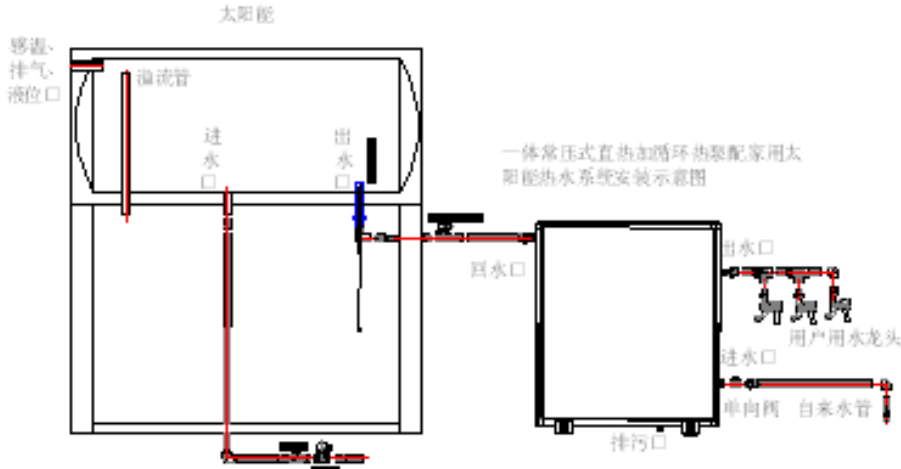
家用一体机与太阳能安装管道连接简图三：
