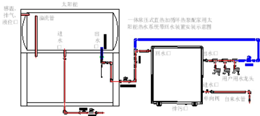
家用一体机与太阳能安装管道连接简图三：
