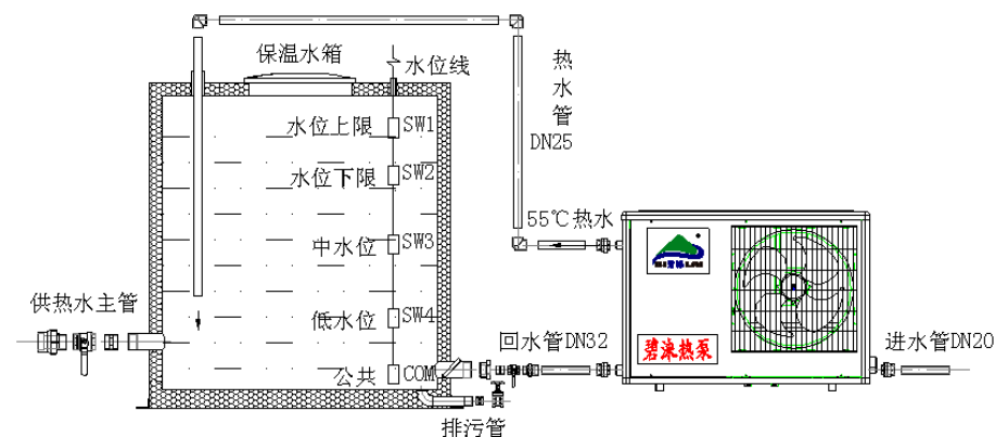
家用分体机管道连接简图二：
