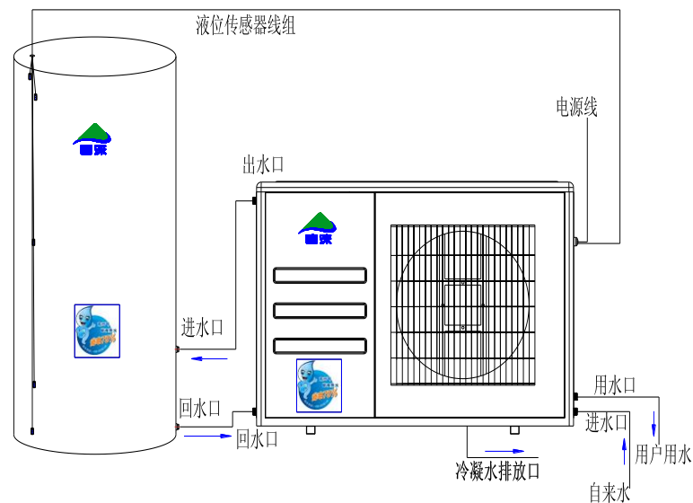
家用分体机管道连接简图二：
